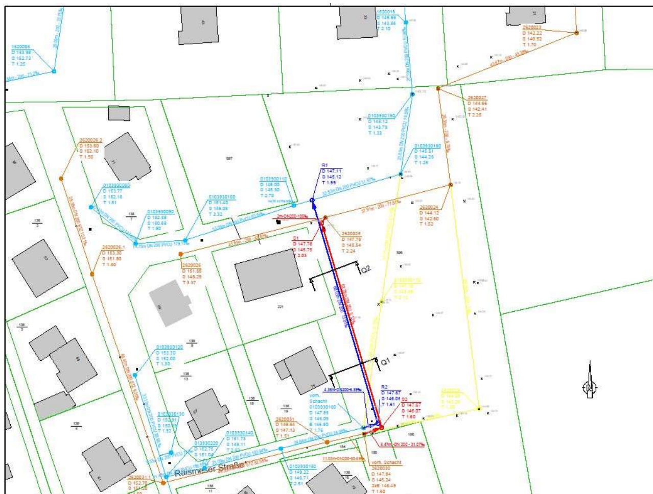
Foto 1: Leitungsbestandsplan
