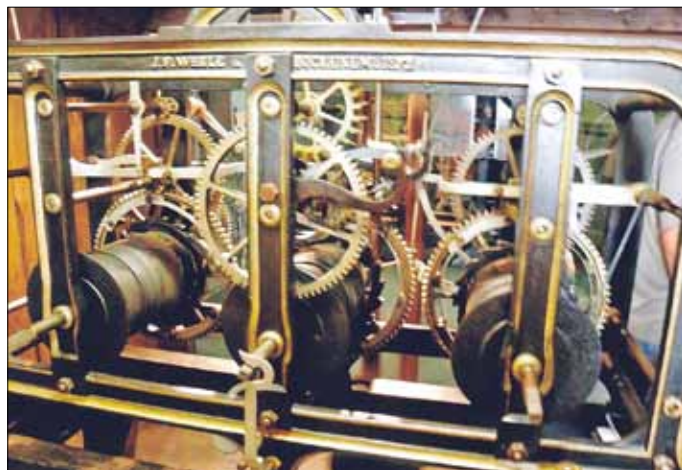
Das „neue“ Uhrwerk der Fa. Weule, Bockenem a. Harz, geliefert 1877 für den Standort St.-Andreas- Kirche
